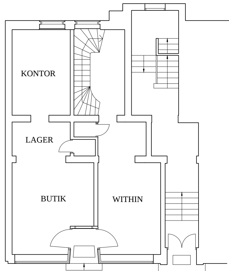
BOTTENVÅNING
