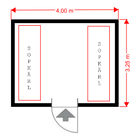
PLAN RITNING Miljöhus
