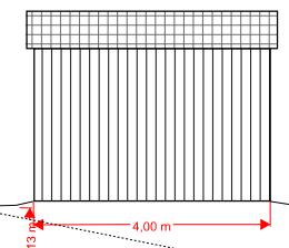
FASAD MOT NORDÖST Miljöhus
