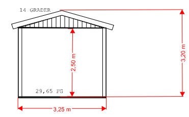
SEKTIONS RITNING Miljöhus
