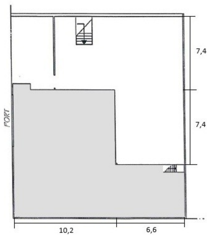
Entresolplan
