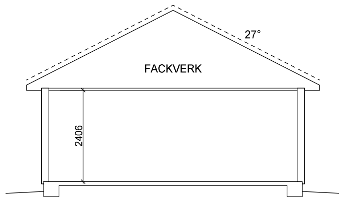
SEKTION A - A
