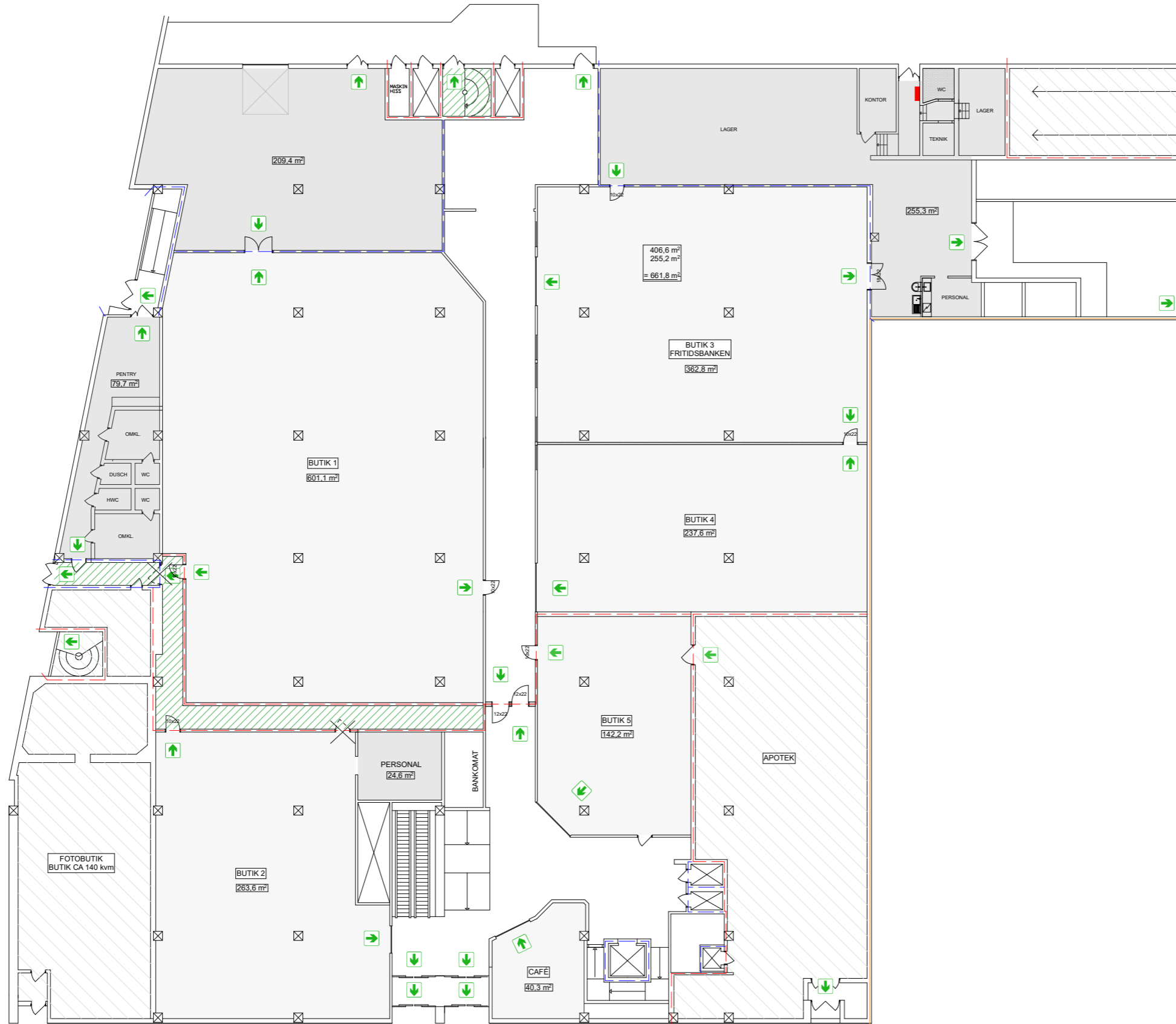
PLAN 1 - ENTRÉPLAN
