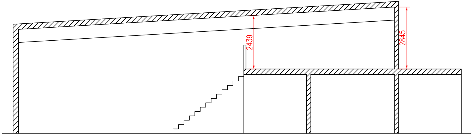
Sektion A-A
