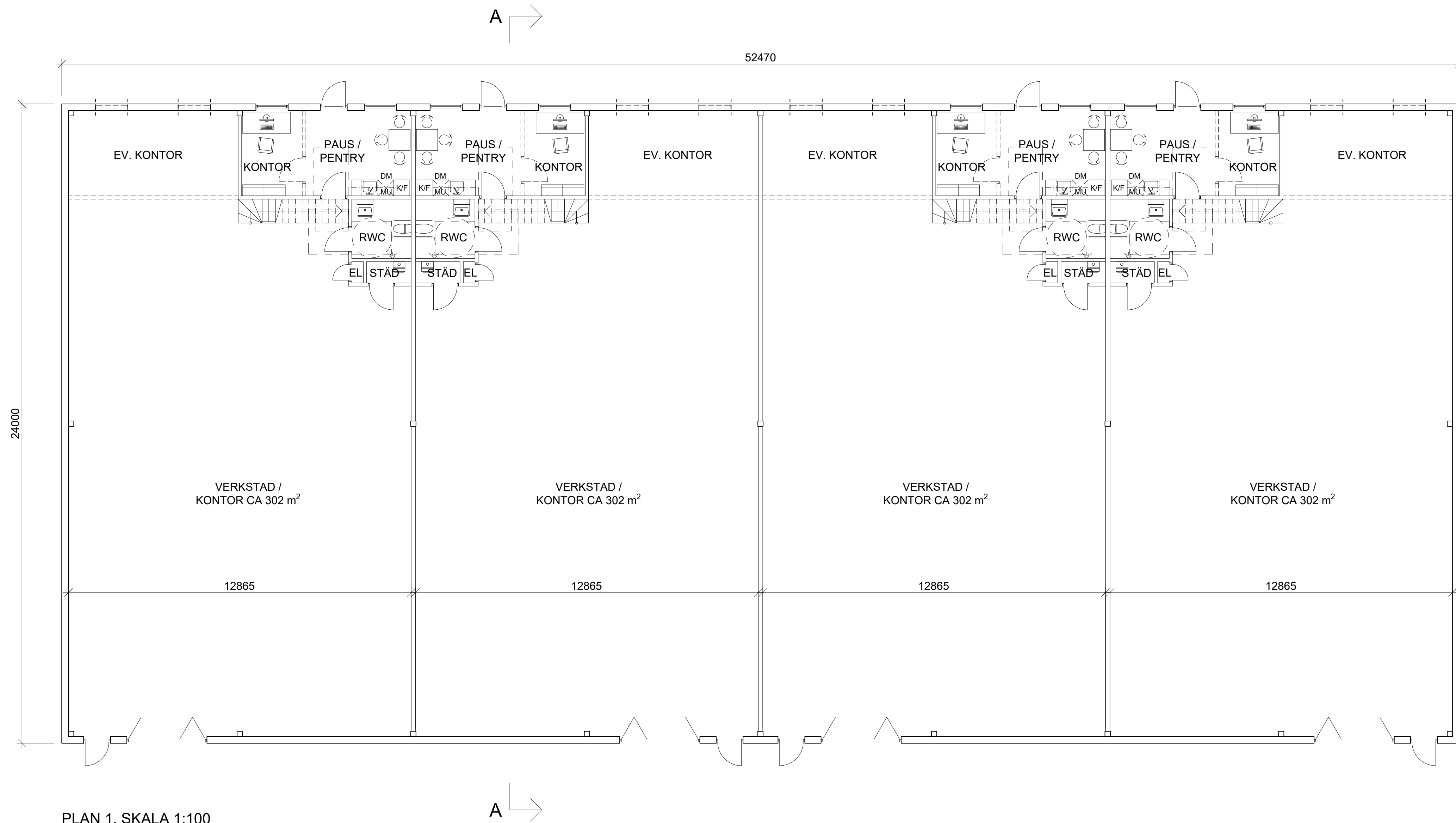
PLAN 1, SKALA 1:100
