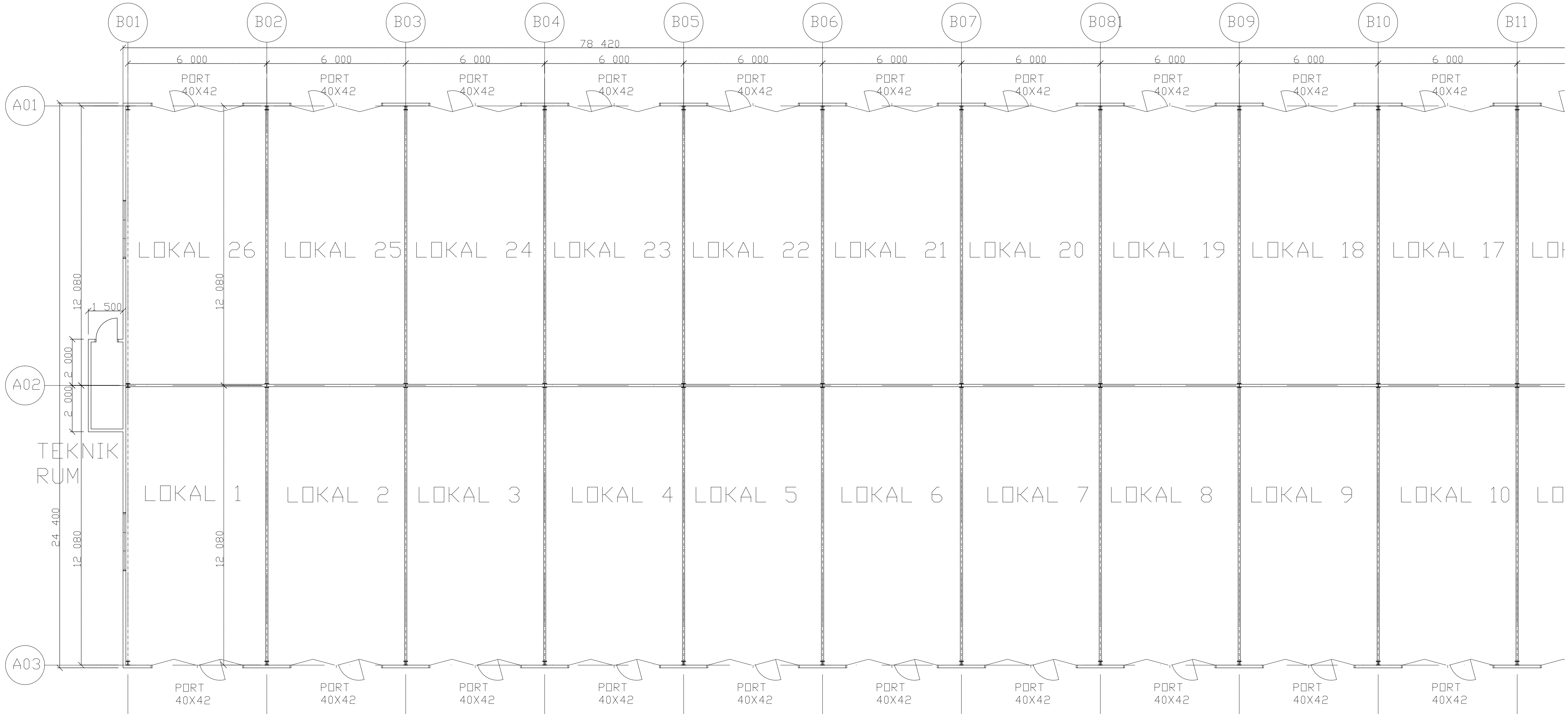
VÄNINGSPLAN
