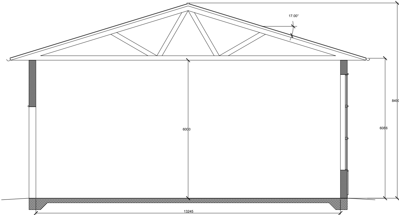
Sektion A-A
