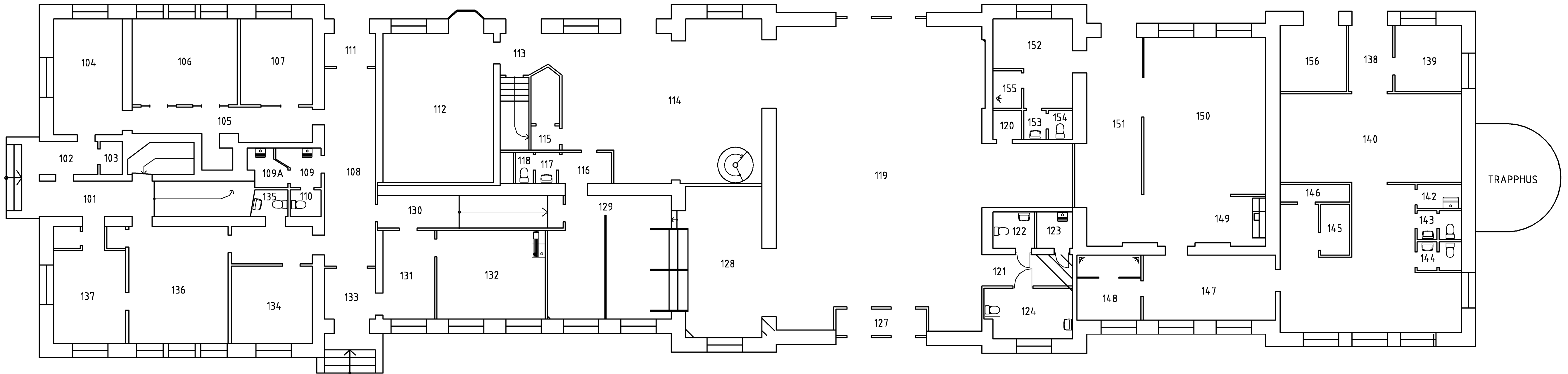
PLAN. BOTTENVÅNING
