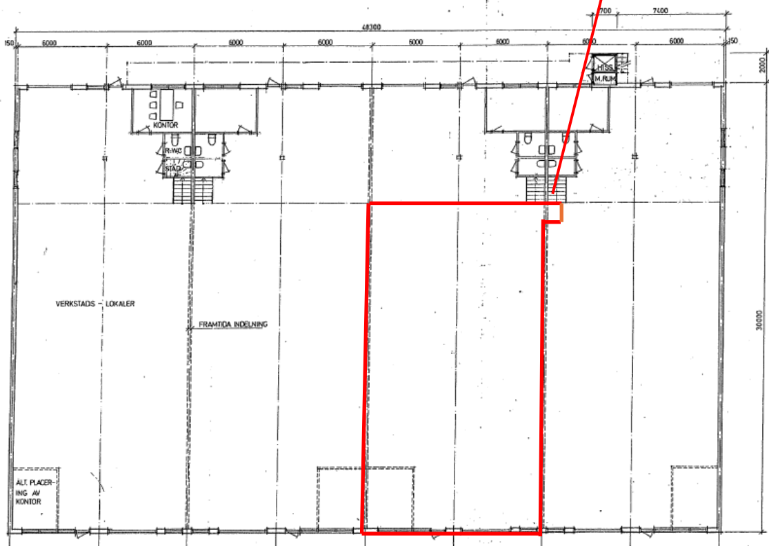
BOTTENPLAN 1:100
