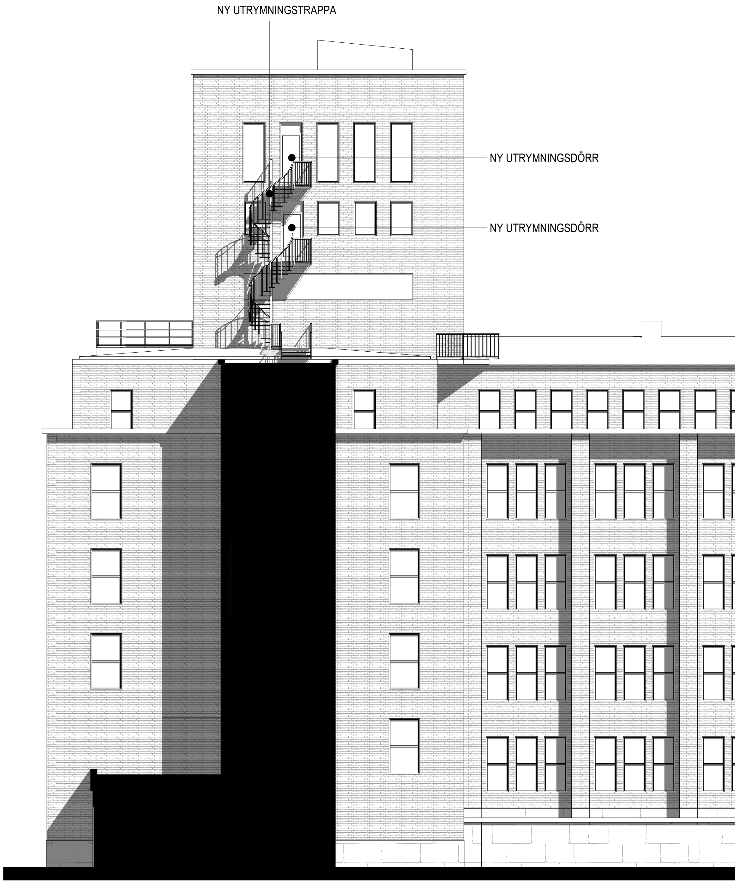
FASAD MOT NORR 1:100
