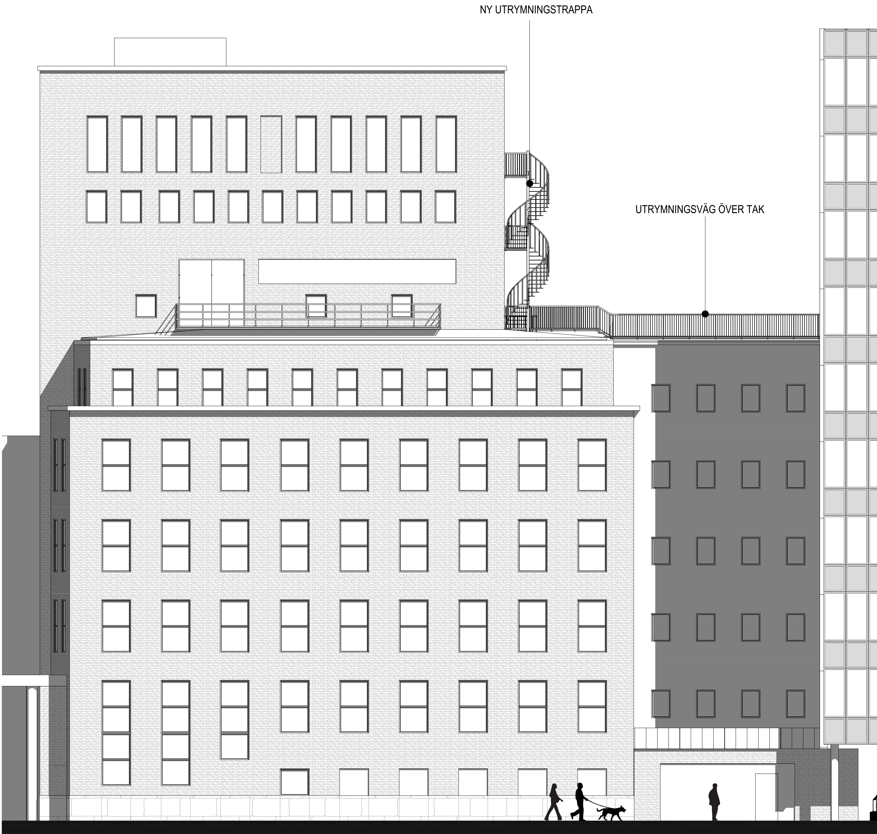
FASAD MOT ÖSTER 1:100
