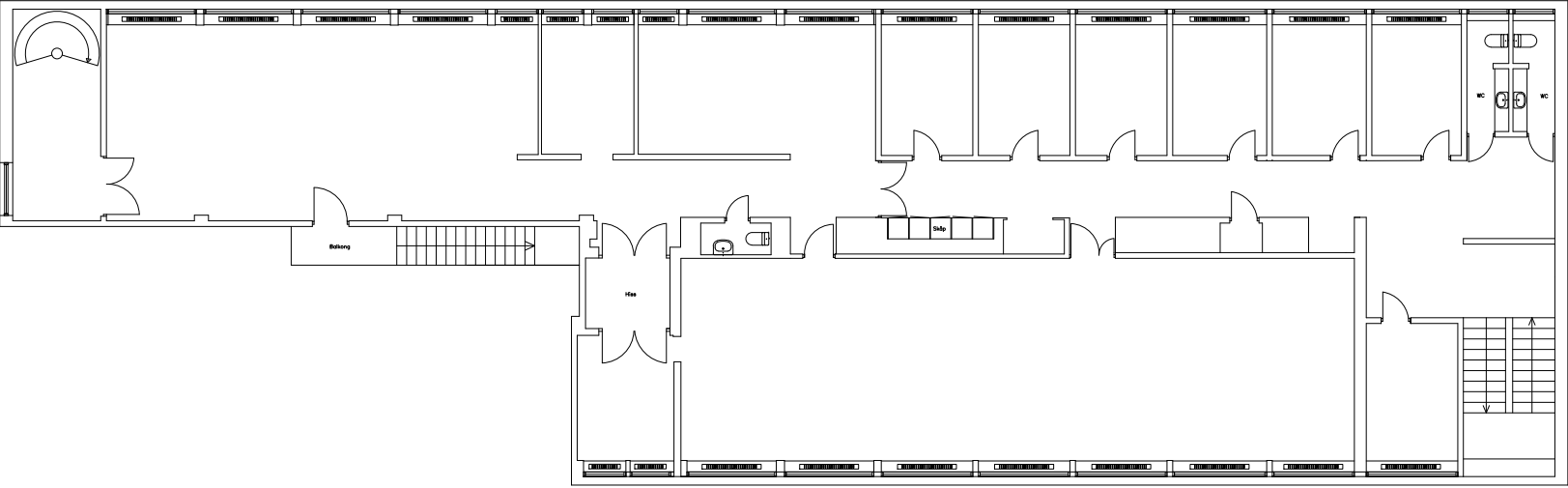
Våningsplan 1
