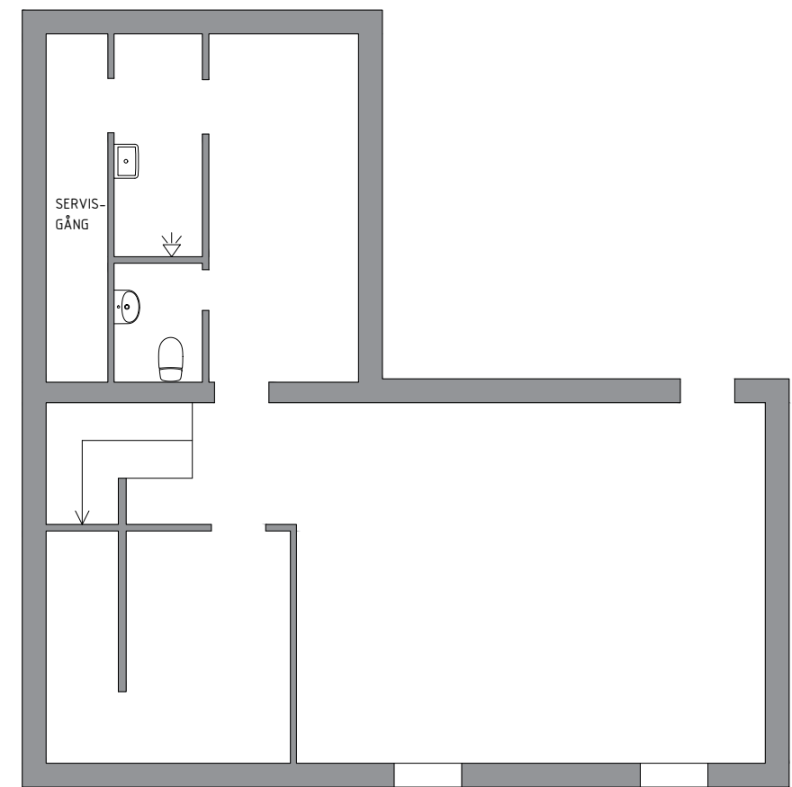
KÄLLARPLAN
