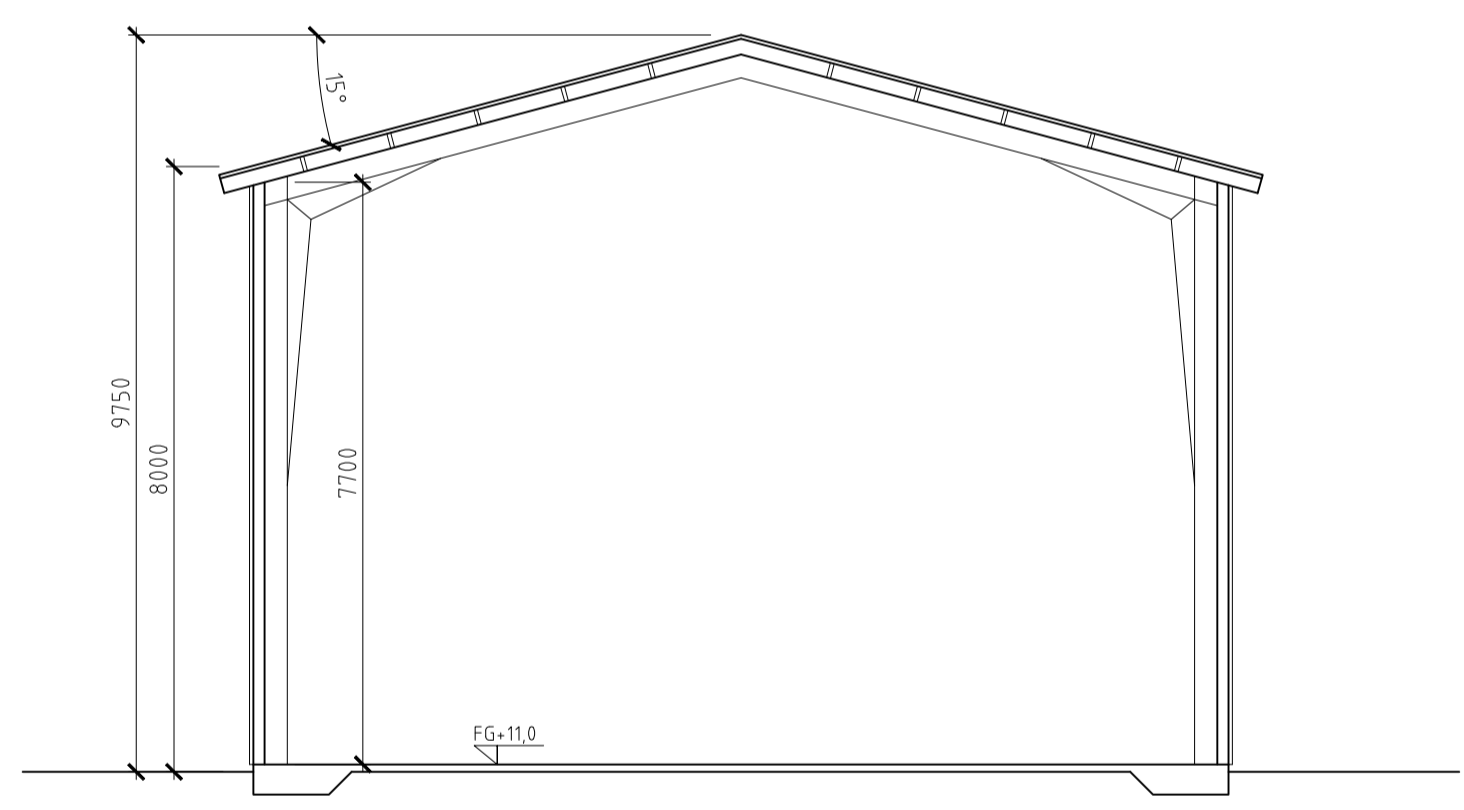
SEKTION A-A
