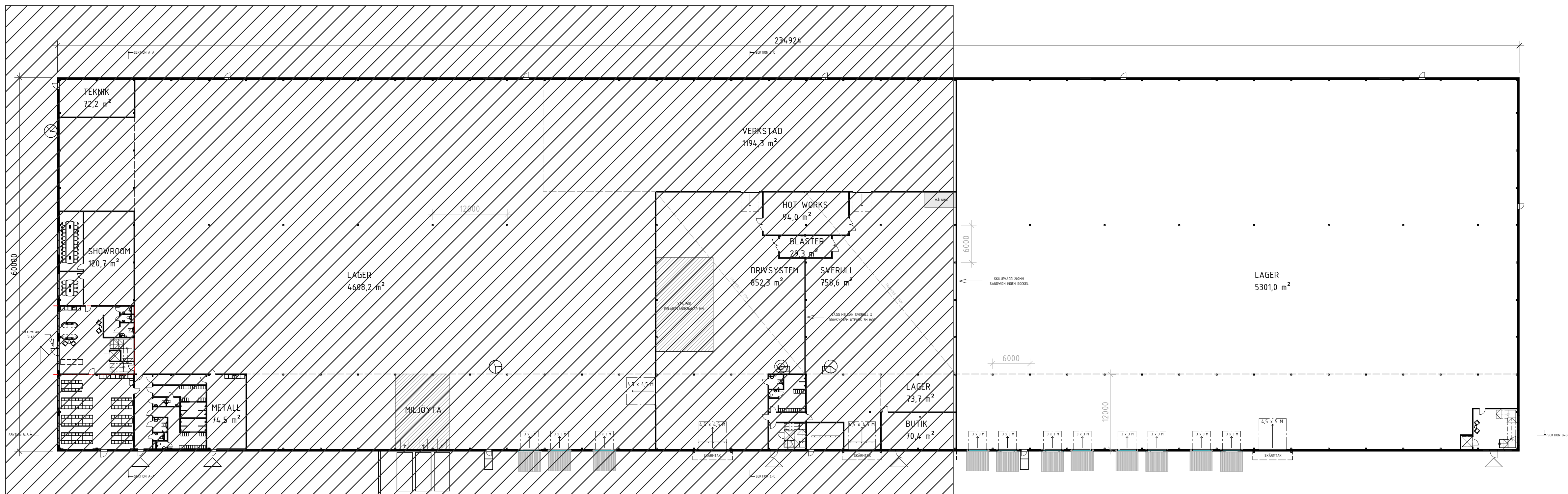
PLAN 1 1 : 400
