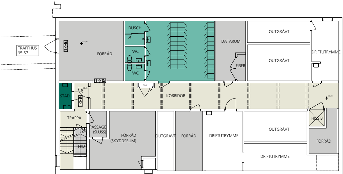
PLAN 1 - KÄLLARPLAN
