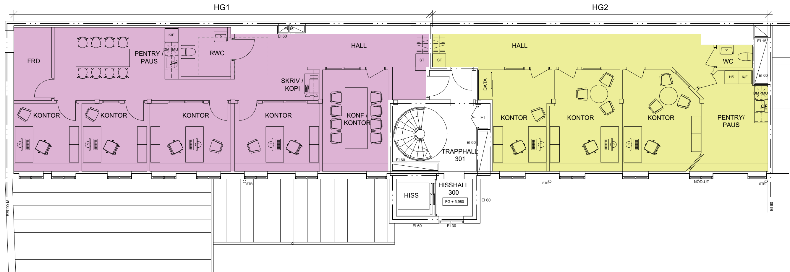
PLAN - VÅNING 3
